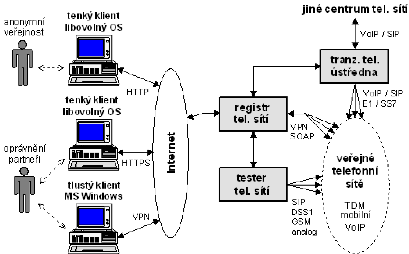
Obr. 1 - Logické schéma centra telefonních sítí
