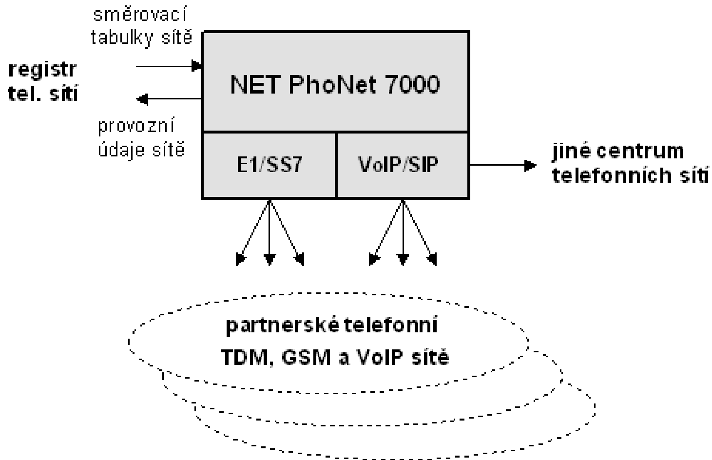
Obr. 4 - Logické schéma tranzitní telefonní ústředny
